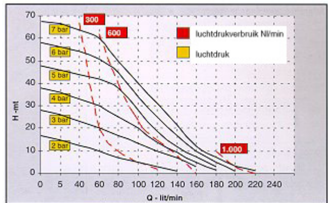
Capaciteit, druk en luchtverbruik Indien uitgevoerd met membranen in PTFE neemt de capaciteit met ca 15% af
