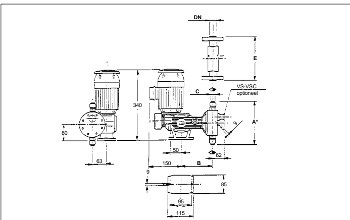
maatschets van de MRB-serie
